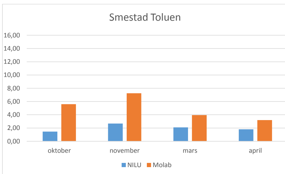
Figur 6. Parallelle målinger for toluen høsten 2013 og våren 2014 ved Smestad
