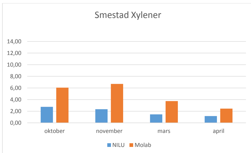
Figur 10. Parallelle målinger for xylener høsten 2013 og våren 2014 ved Smestad
