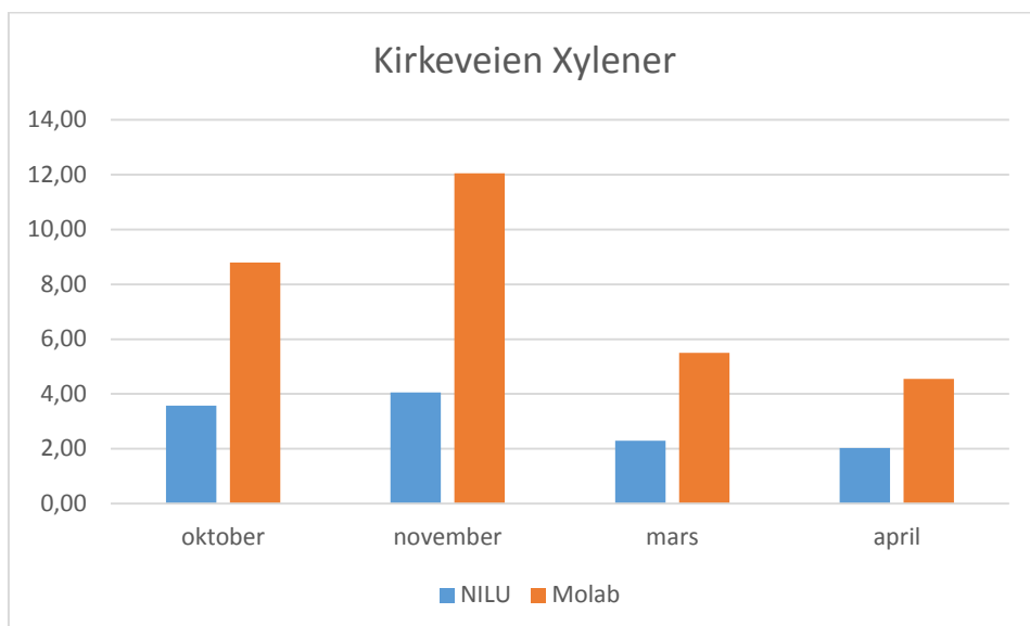
Figur 9. Parallelle målinger for xylener høsten 2013 og våren 2014 i Kirkeveien
